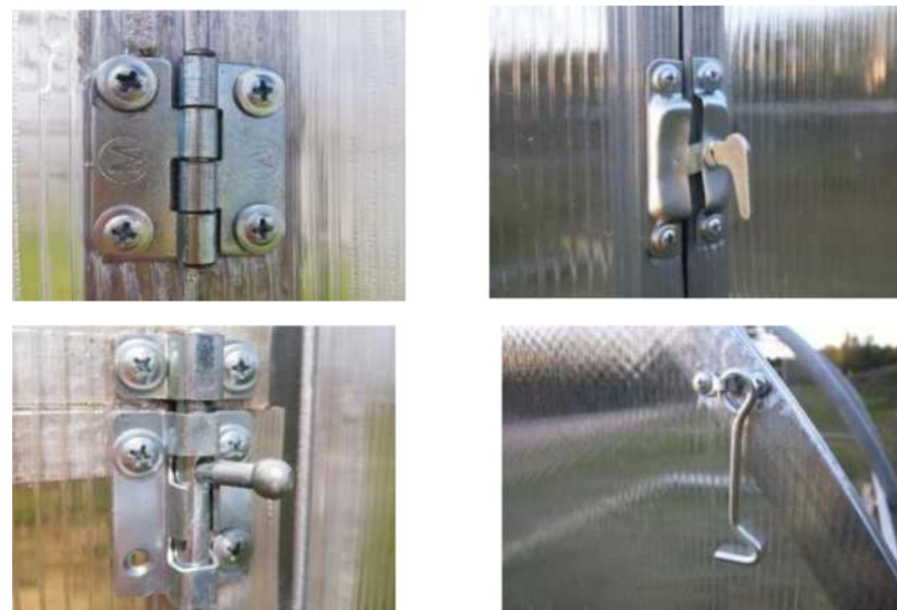
Pav. 2.2 – Lankstų, suktuko, skląščio, kabliuko tvirtinimas
