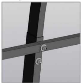
Pav. 3.1 – Lankų ir skersinių tvirtinimas šiltnamio viduje
